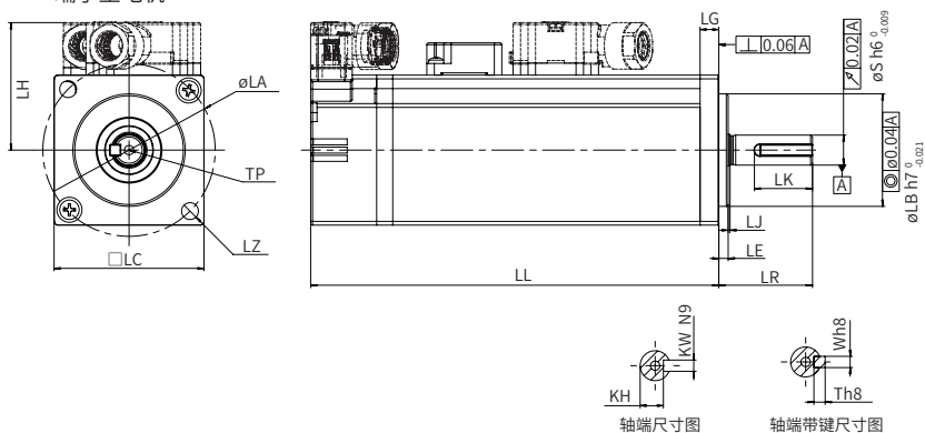
轴端尺寸图
