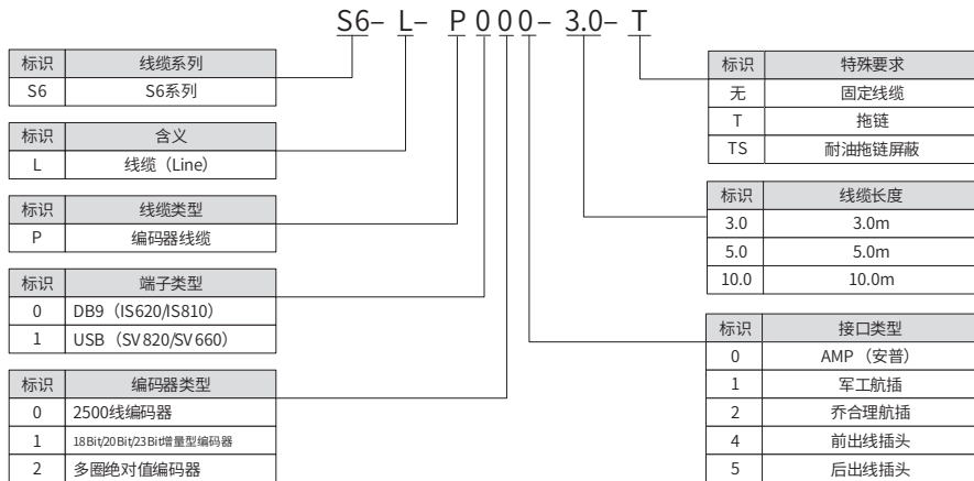
图 3-1 编码器线缆型号说明
