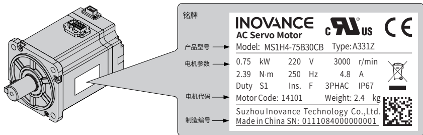
图 1-1 电机型号与铭牌信息
