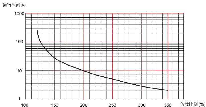
图 1-6 电机过载曲线
