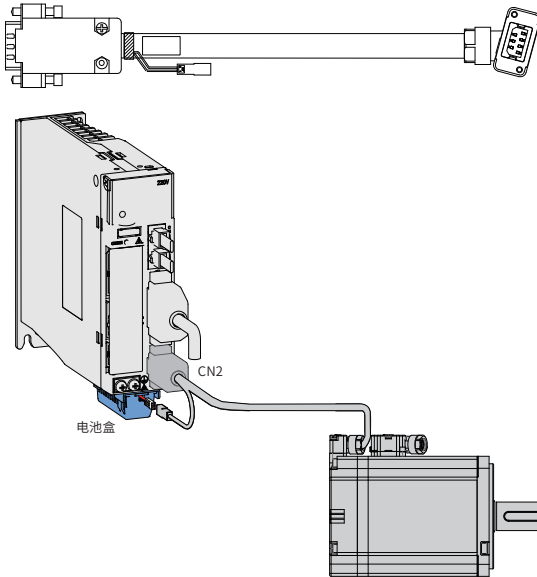
图 3-9 与 IS620 系列伺服驱动器编码器线连接示意图
