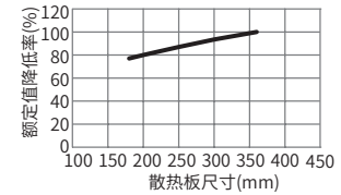
■ 散热降额曲线
