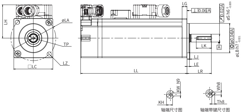
轴端尺寸图
