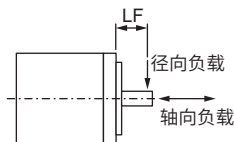
图 2-1 电机径向及轴向载荷示意图
