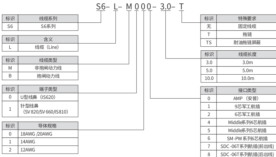
图 3-2 动力线缆型号说明
