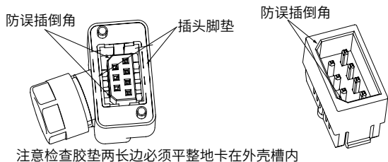
图 3-16 编码器连接器
