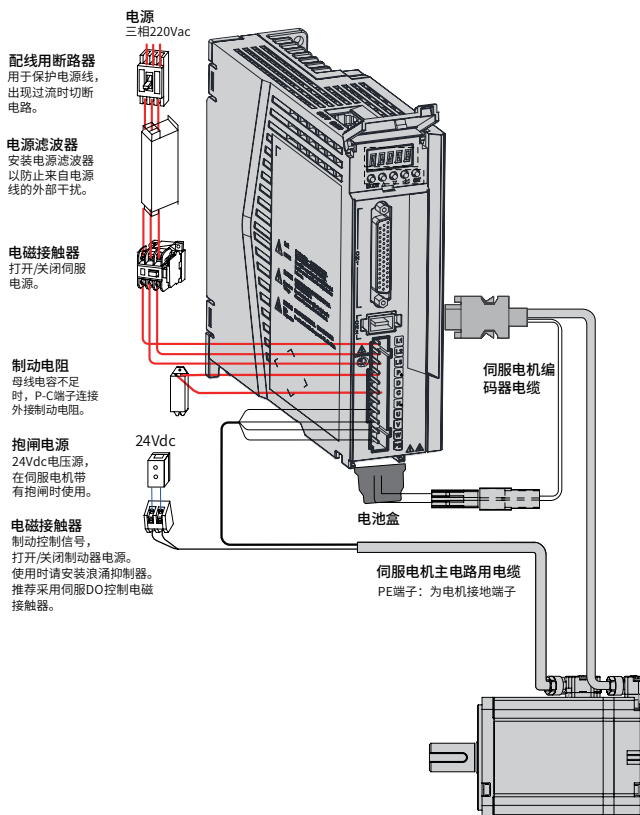
图 1-5 系统构成
